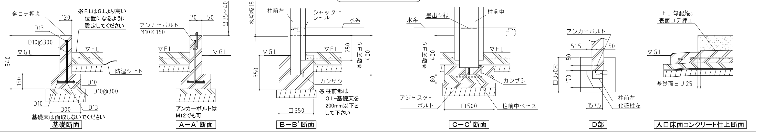
基礎図 <縮尺> S=1/50 ~一般型~
